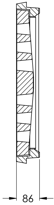
SECTION A-A
